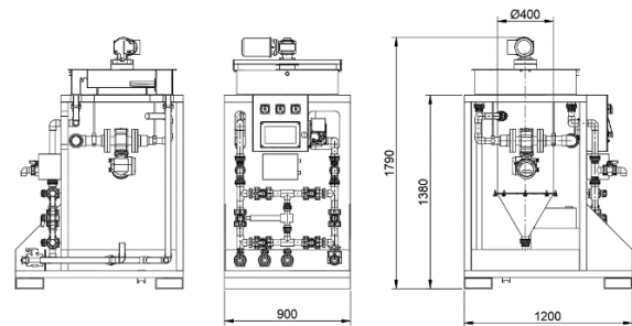
Abmessungen des PreSep [trial]
