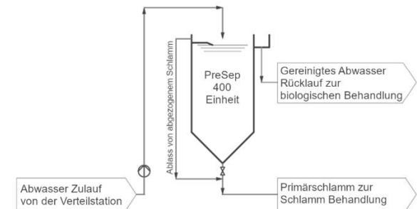
Prozess-Schema des PreSep [trial]
